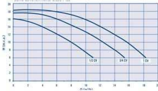
Courbes de débit
